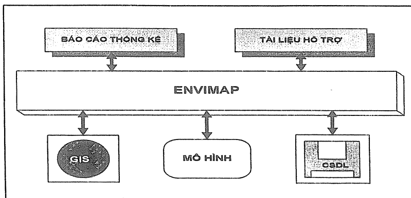
Hình 1. Sơ đồ cấu trúc (các module) của phần mềm ENVIMAP
