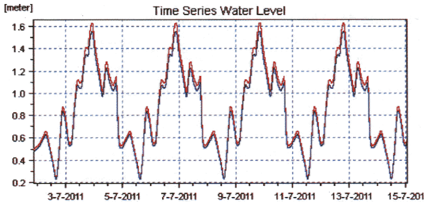
Hình 5. So sánh kết quả kiểm định mô hình thủy lực tại trạm Đập Truồi 1/7 – 15/7 2011.
