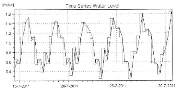
Hình 4. So sánh mực nước giữa kết quả tính toán và số liệu mực nước thực đo tại các trạm Cầu Máng (trái) và Đập Truồi 1 (phải) từ 15/7/2011 tới 30/7/2011
